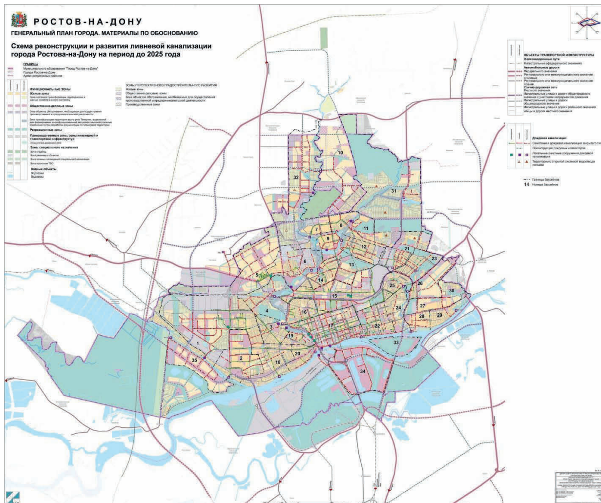
Рис. 3. Водосборные бассейны схемы ливневой канализации
